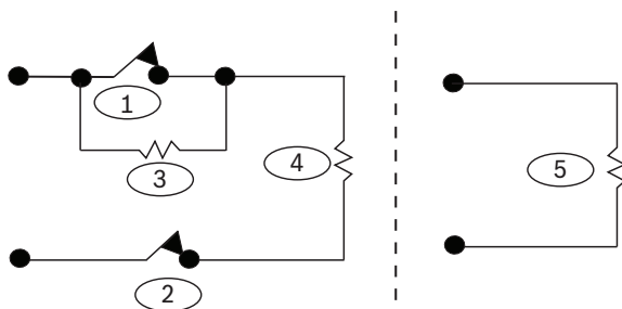
Σχήμα 12.1: Επιλογή διπλής αντίστασης τερματισμού γραμμής
