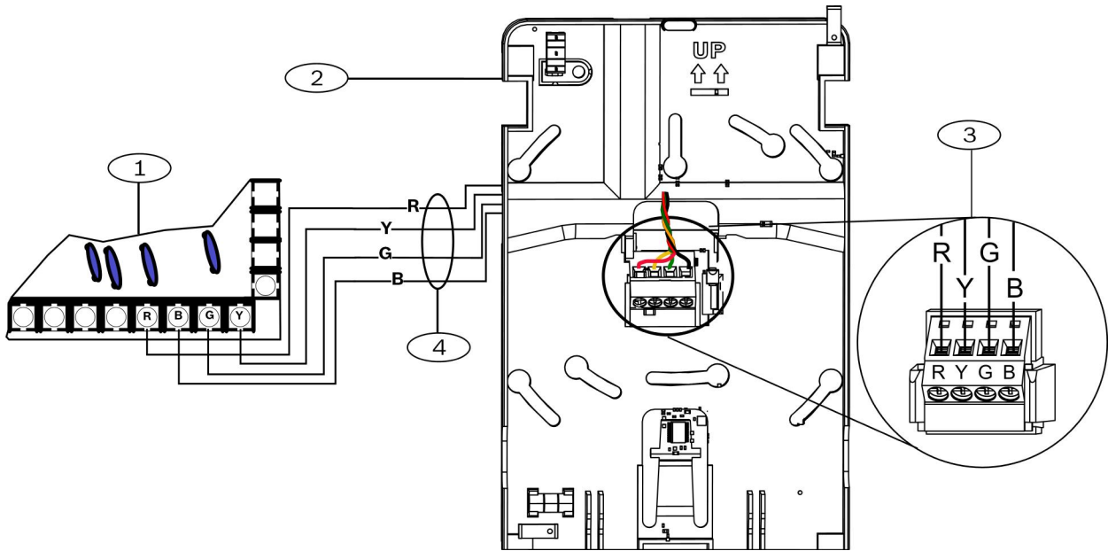
Σχήμα 3.1: Καλωδίωση κλεμοσειράς ακροδεκτών σε δίαυλο επιλογής
